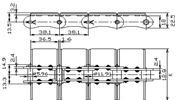
TPW形
