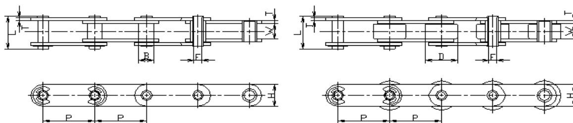
チェーン各部寸法
