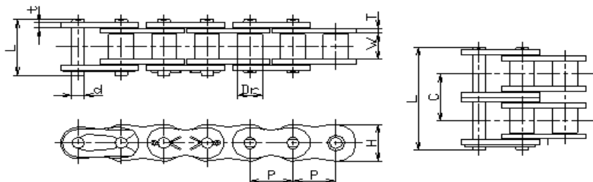
チェーン各部寸法
