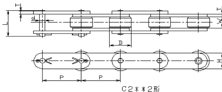
チェーン各部寸法
